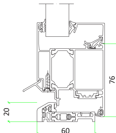
Porte-fenêtre sur seuil
