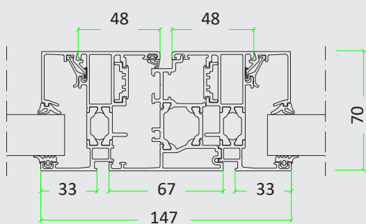
Battement central fenêtre
