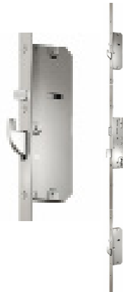
Serrure 3 pènes à crochets
