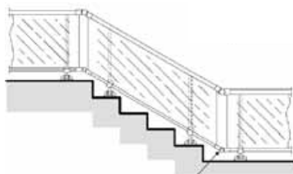
Rampant pose sur dalle
