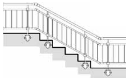
Rampant pose à l'anglaise
